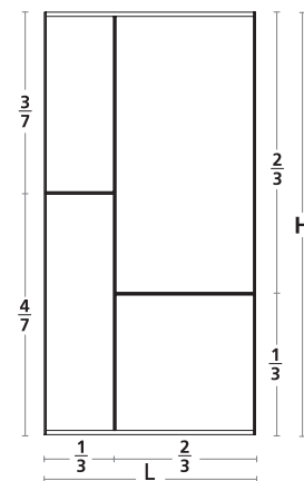
codice code SPO2P04
