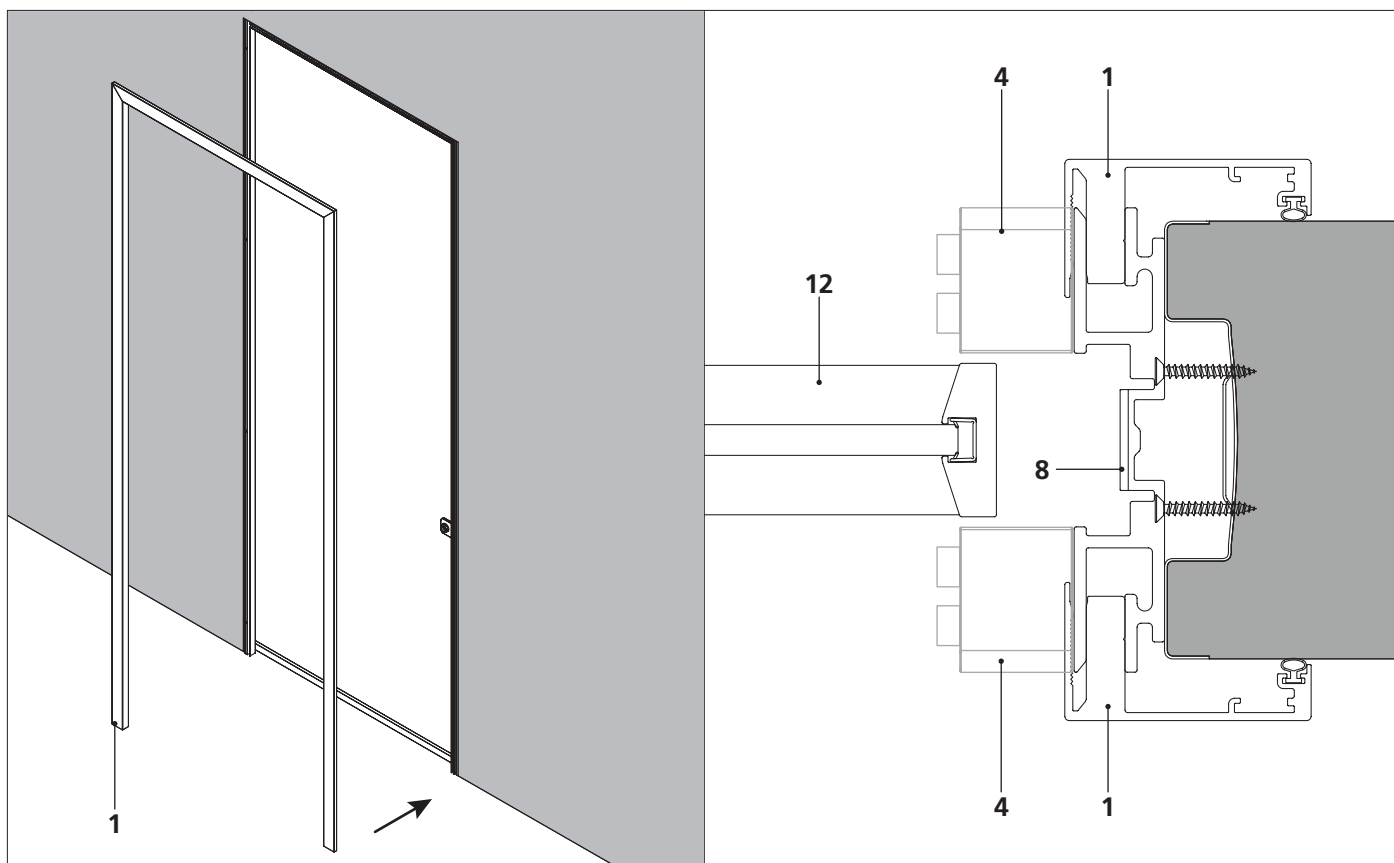
Posizione dello stipite esterno External jamb's position.
