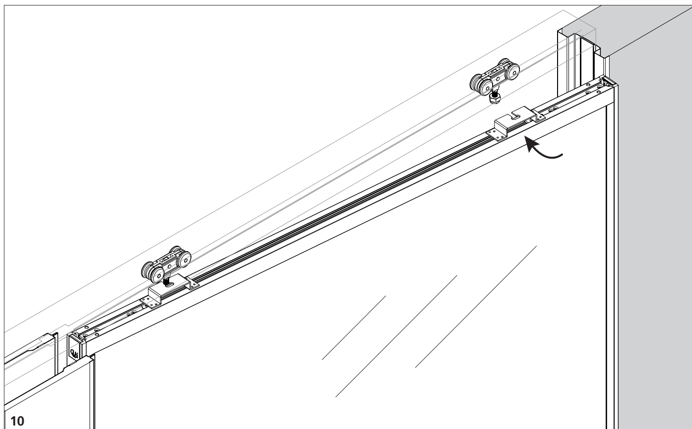
10. Appendere l'anta al secondo carrello. 10. Hang the door on the second carriage.
